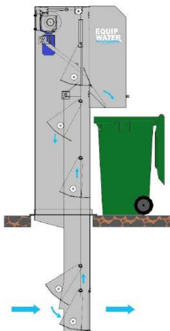
Fonctionnement Dégrilleur Vertical XS
